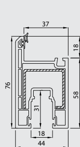
Super Sash Profile(I-64) 41164-20300
