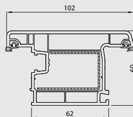
Door Sash Profile 41101 - 14000
