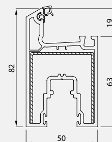
Sash Profile(I-64) 41164-20100
