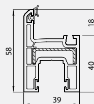
Sash Profile(I-60) 41201 - 03300
