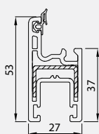
Sliding Sash(I-44) 41231-13100
