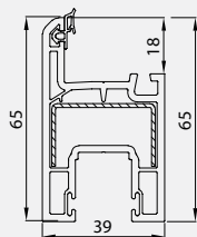
65mm Sash Profile(I-60) 41201 -03200
