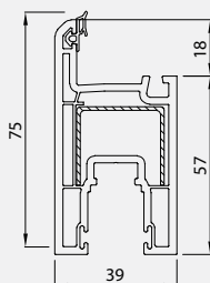
Super Sash Profile(I-60) 41201 - 03000
