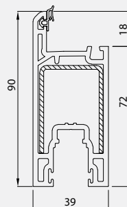
Mega Sash Profile(I-60) 41201 - 07000
