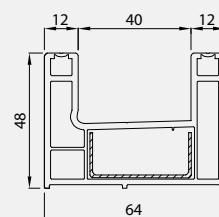
Double Rail Profile(I-64) 41164-10100
