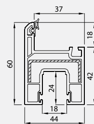
Sash Profile(I-64) 41164-20100
