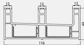
Triple Rail Profile(I-64) 41264-10300
