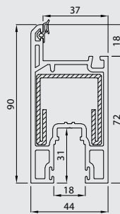
Mega Sash Profile(I-64) 41264-20400
